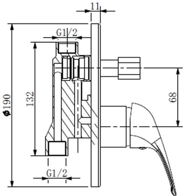
A-A Scale 0.300
